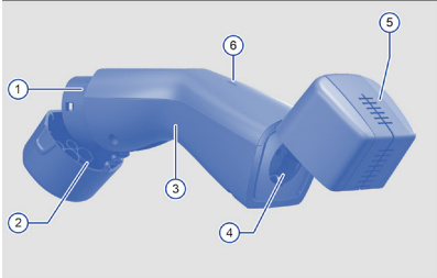
Fig.1 Harsa Ġenerali lejn il-PowerSocket
