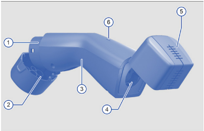
그림 1 파워소켓 개요
