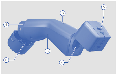
Fig. 1 Oversigt PowerSocket
