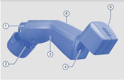
Fig. 1 Visione generale PowerSocket
